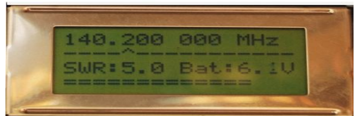
Sistemul de afișaj al SWR realizat de HG7AC
