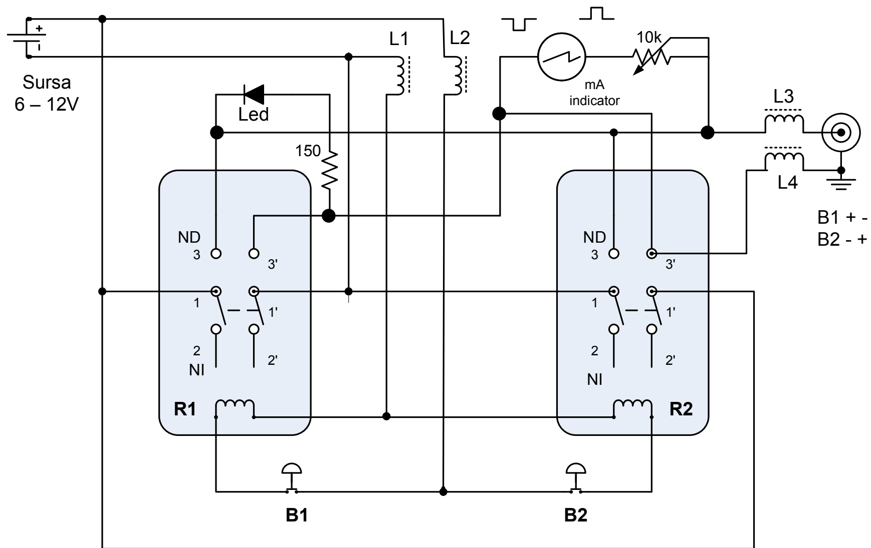
Alimentare cu inversor de polaritate pentru motor de curent continuu
